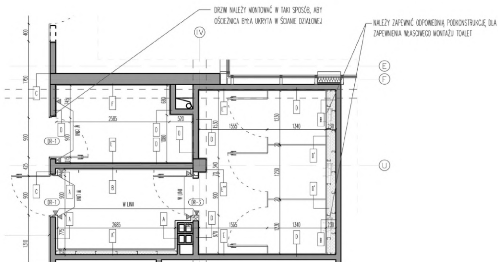
PLAN KONSTRUKCYJNY
