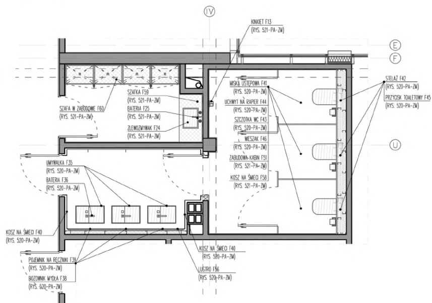
PLAN ARANŻACJI
